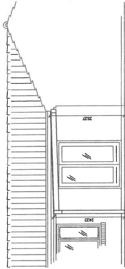
Snit i overdækning i gårdrum
