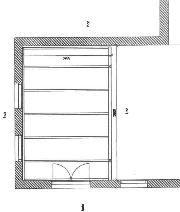
Plan af overdækning i gårdrum
